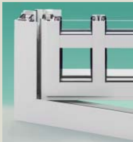
Echte Sprosse glastrennend Typ G 37 37 mm Ansichtsbreite
